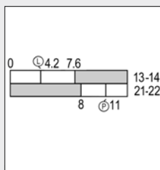
Изображение контуров: Предохранительный концевой выключатель, компактный
