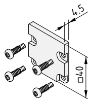
Заглушка для направляющего профиля 8 40x40
