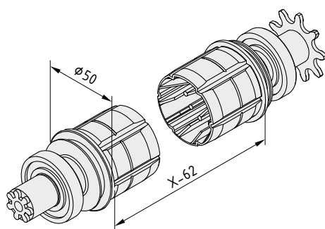
Комплект приводных подшипников для конвейерного ролика TRA50 (с цепным приводом)
