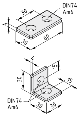
Кронштейн 6 30 плоский
