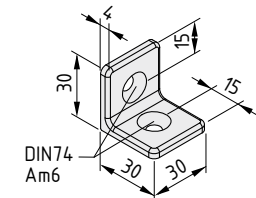
Угловой кронштейн 6 30 прямоугольный
