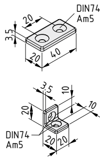
Кронштейн 5 20 плоский
