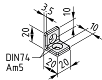
Угловой кронштейн 5 20 прямоугольный
