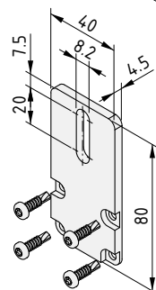
Заглушка для направляющего профиля 8 80x40
