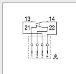
Схема соединений: Предохранительный концевой выключатель, компактный
