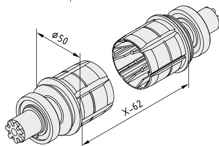
Комплект подшипников для конвейерного ролика TRA50 (с цепным приводом)
