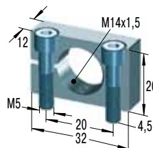
Опора-зажим
