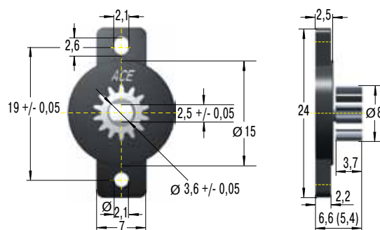
FRT-G2 (при 23 °C)
