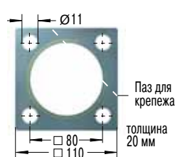
Квадратный фланец
