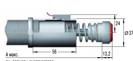
Ограничительная втулка
