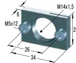
Прямоугольный фланец
