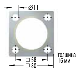
Квадратный фланец
