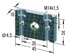
Универсальная опора
