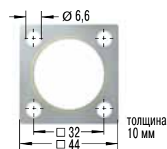
Квадратный фланец
