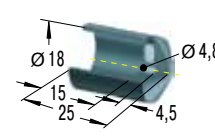
Защитный колпачок
