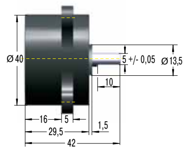
FRT-K2 и -F2 (при 20 об/мин)
