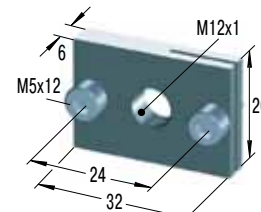
Прямоугольный фланец
