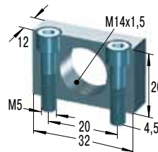
Монтажная опора
