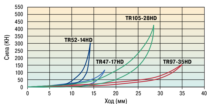
График "Усилие - Длина хода" (статическая характеристика)
