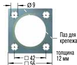
Квадратный фланец
